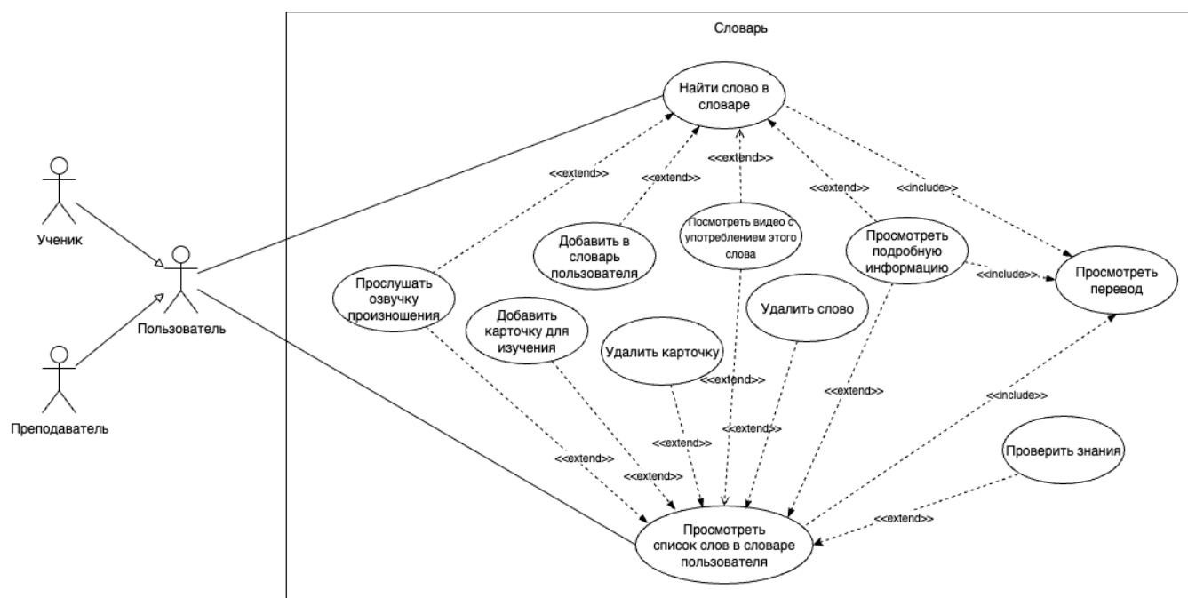
Рисунок 2. Диаграмма Use Case для версии 2.0 веб-приложения Chatty
